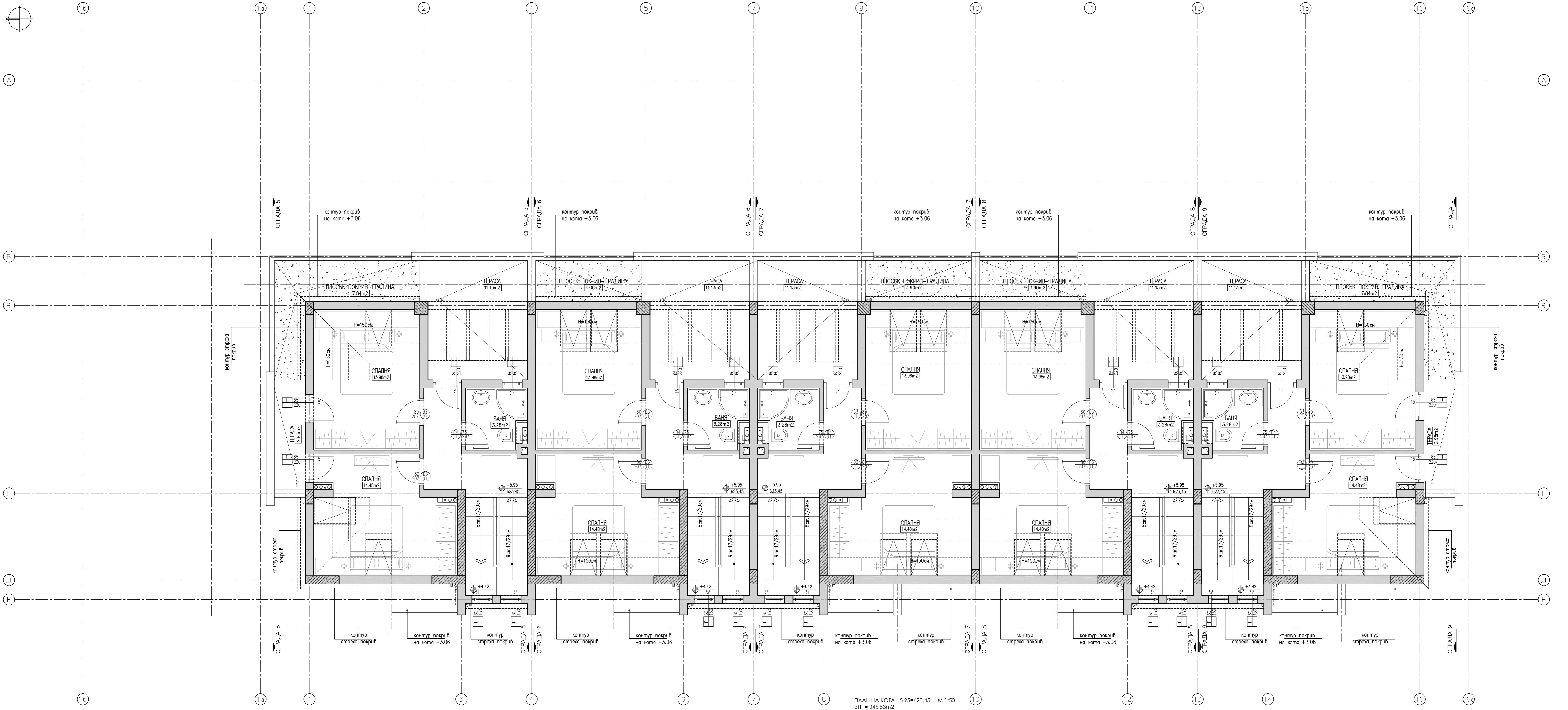
СГРАДА 5 ПЛАН НА КОТА +5.95=623.45 М 1:50 ЗП = 75.64м2
